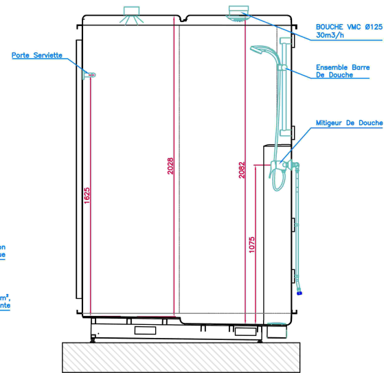
ELEVATION C-C
