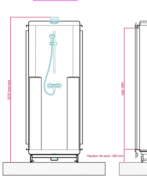
ELEVATION A-A
