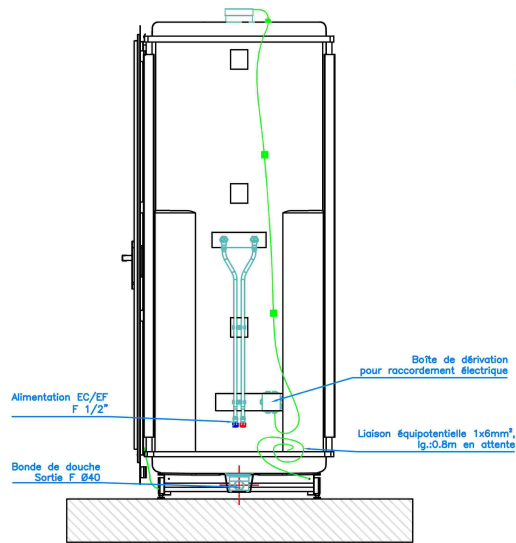
VUE SUIVANT B
