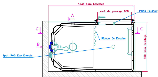
ENCOMBREMENT SUIVANT SENS 01 ET 02
