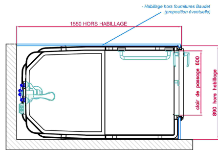
ENCOMBREMENT SUIVANT SENS 03 ET 04
