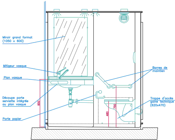
ELEVATION A-A
