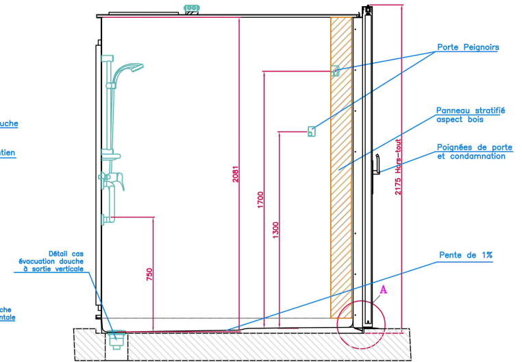
ELEVATION B-B (version avec décaissé)
