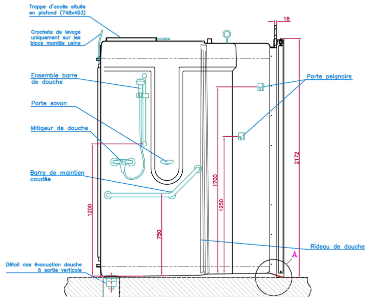
ELEVATION A-A
