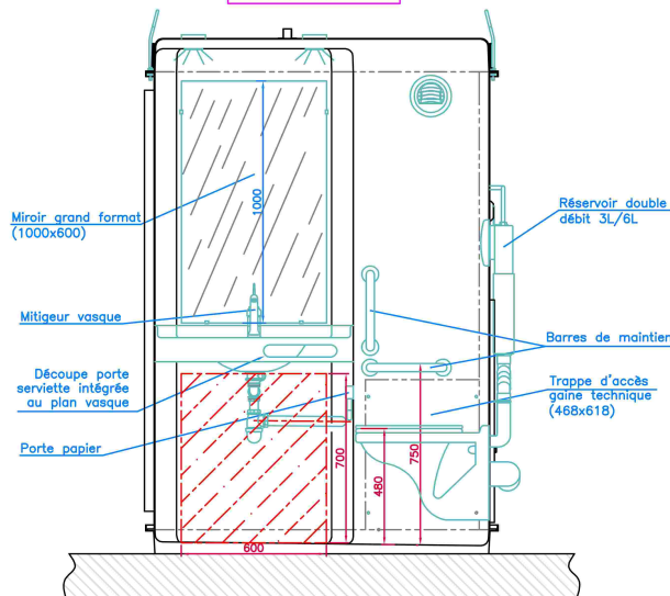
ELEVATION B-B
