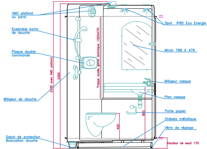
COUPE A-A
