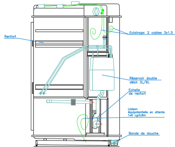
VUE SUIVANT B
