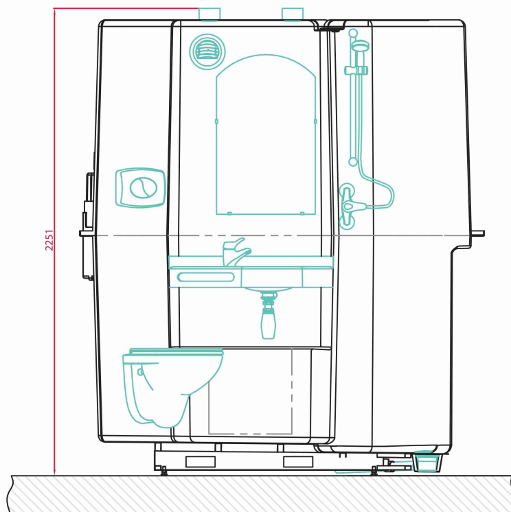
ELEVATION A-A
